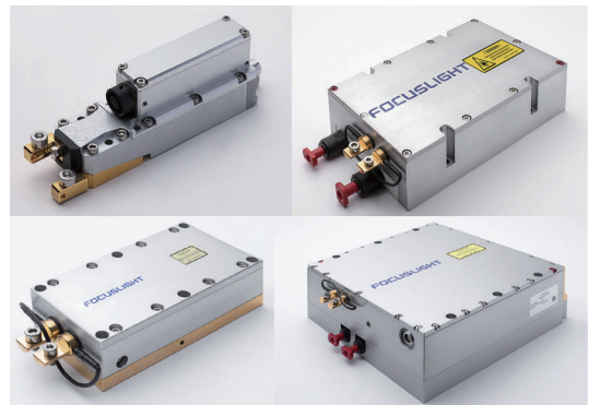
单巴/多巴耦合模块: LM, FG, ND, MF 系列
