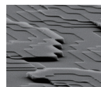
用于深紫外准分子激光光束整形的DOE
