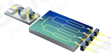
光子集成电路
