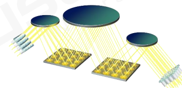
波长选择开关/光路开关
